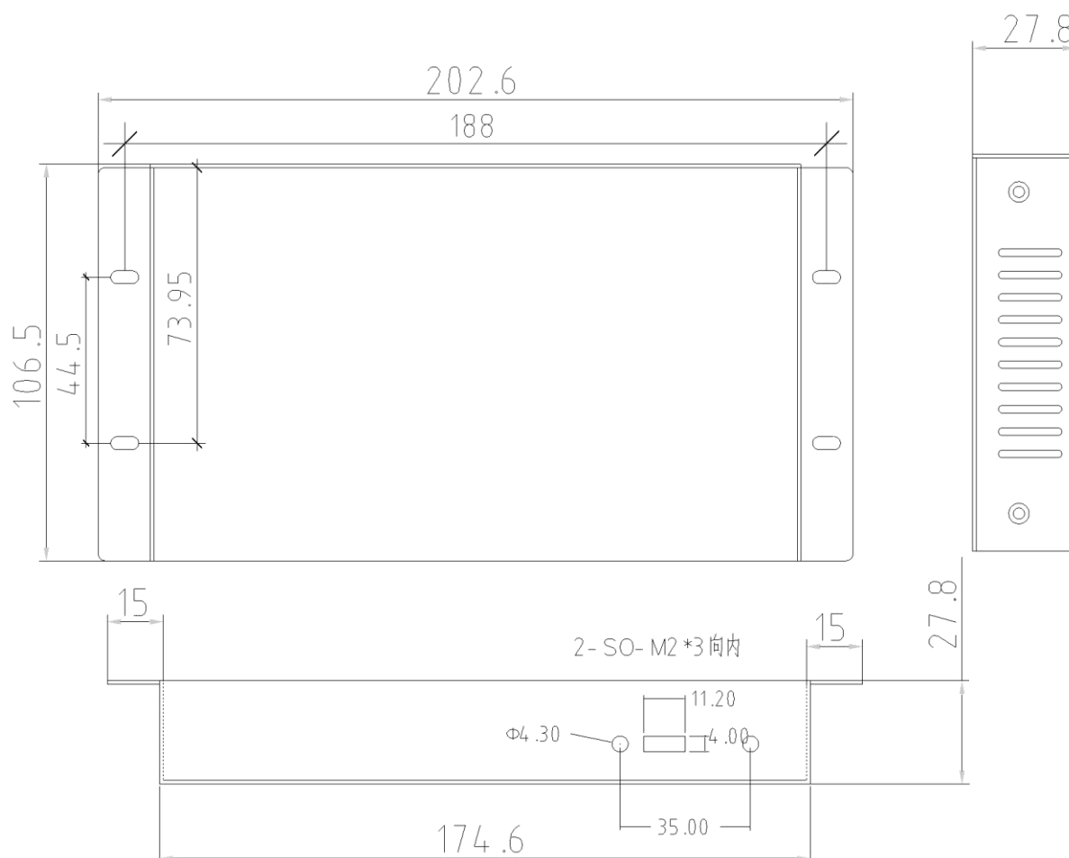
侧面接口尺寸 (装盒)
